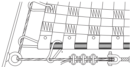
Carabiner Clip w Opt Rod
