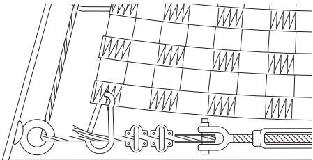
Carabiner Clip w/o Opt Rod
